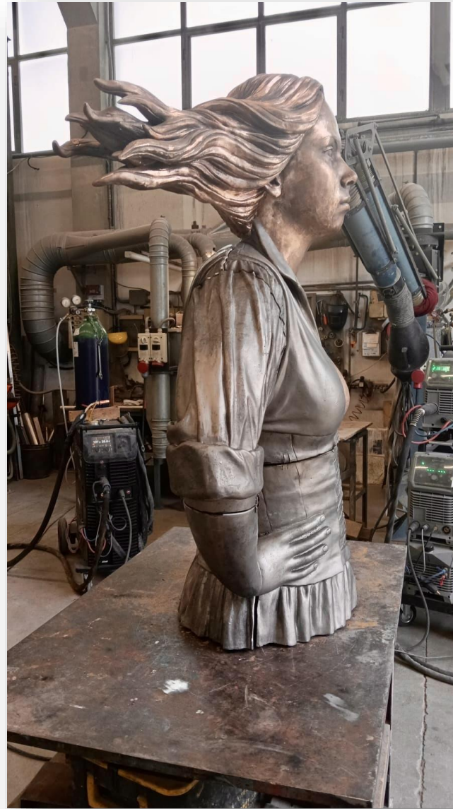
Samenvoegen van de gietstukken
